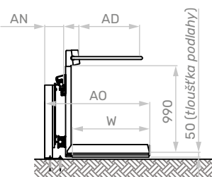
BOČNÍ POHLED OTEVŘENÁ PLOŠINA kotvení na samonosných nohách
