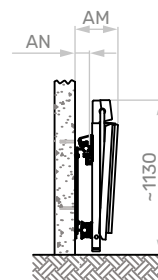
BOČNÍ POHLED ZAVŘENÁ POZICE kotvení na zeď
